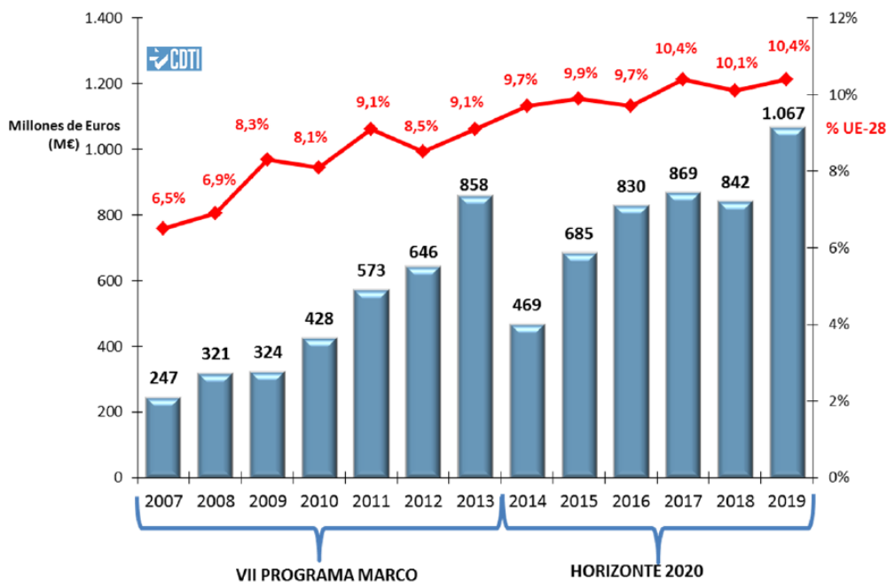
Gráfica 3: Evolución de las cifras de retorno de las entidades españolas en VII PM (2007-2013) y Horizon2020 (2014-
