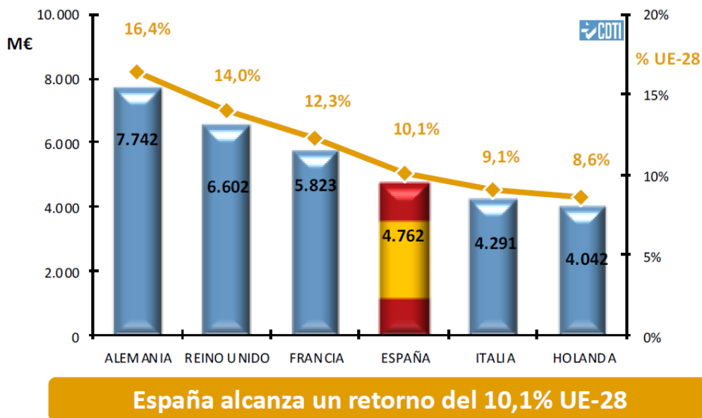
Gráfica 2: Cifras de retorno de las entidades españolas en Horizonte 2020 (2014-2019)
