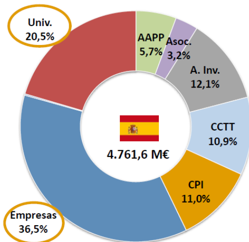
Gráfica 6: Participación española por tipo de entidad.
