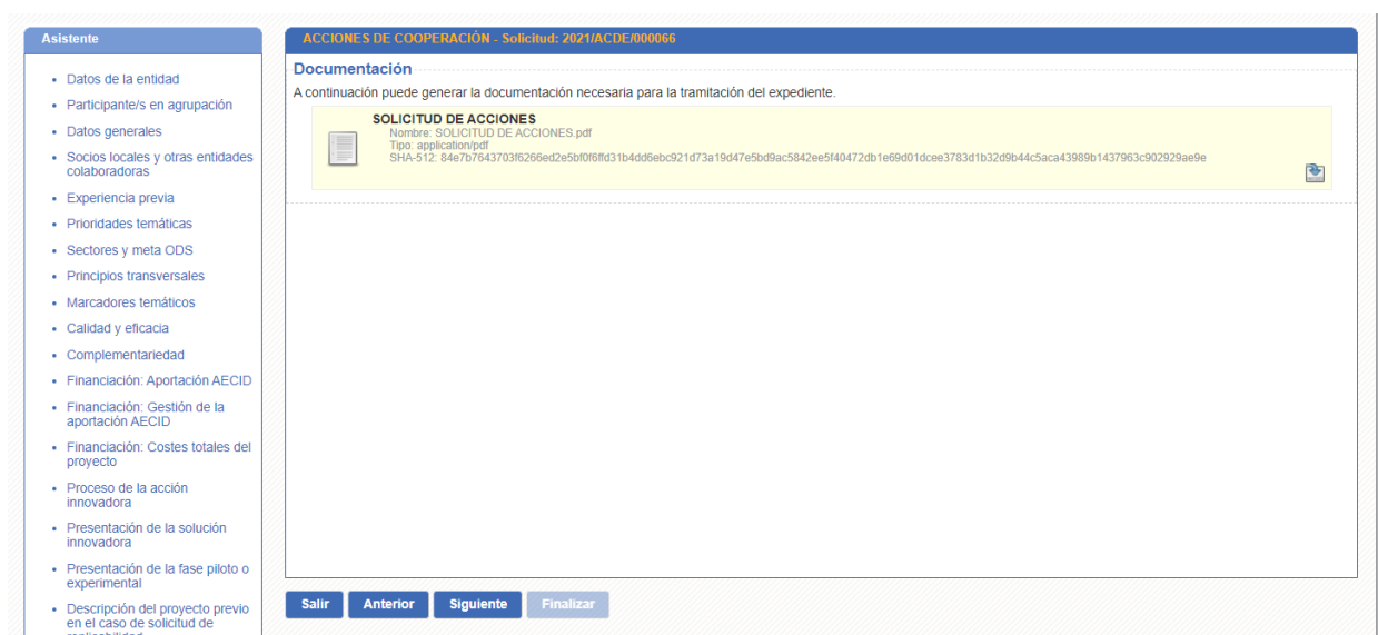
Ilustración 50. Solicitud generada
